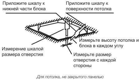
Трафарет для установки
