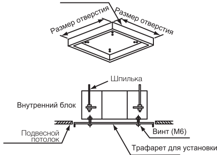
Трафарет для установки
