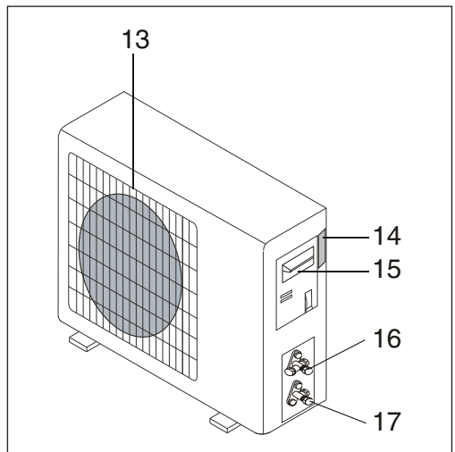
Рис. 3.2. Наружный блок
